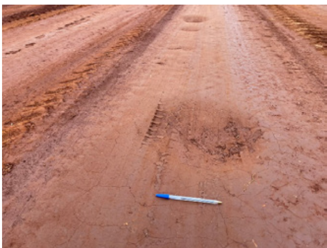
(a) Pequenas panelas e trincas em bloco. Solo com tratamento.
