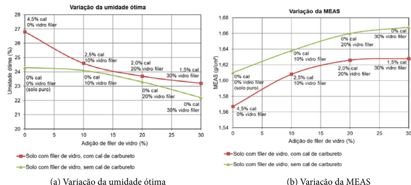
Figura 4: Variação da umidade ótima e da MEAS em função do teor de adição de fíler de vidro nas misturas, com e sem cal de carbureto.
