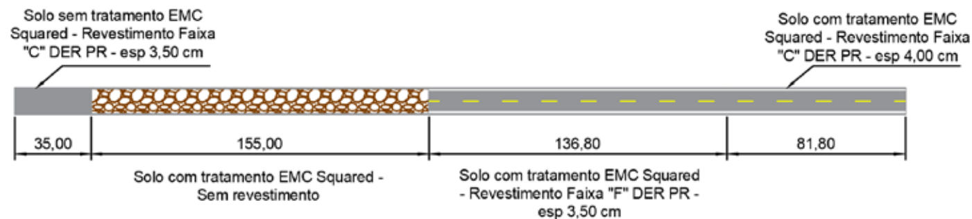
Figura 2: Esquema dos trechos experimentais executados nesta pesquisa.
