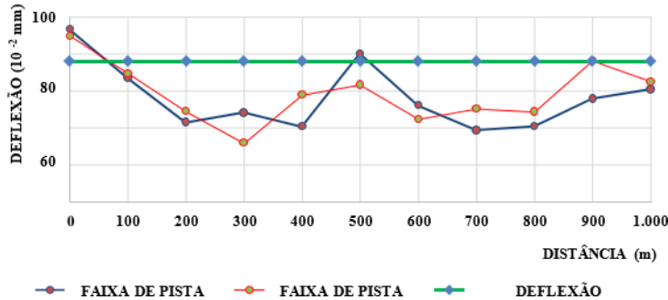
Figura 11: Gráfico de deflexão com viga Benkelman
