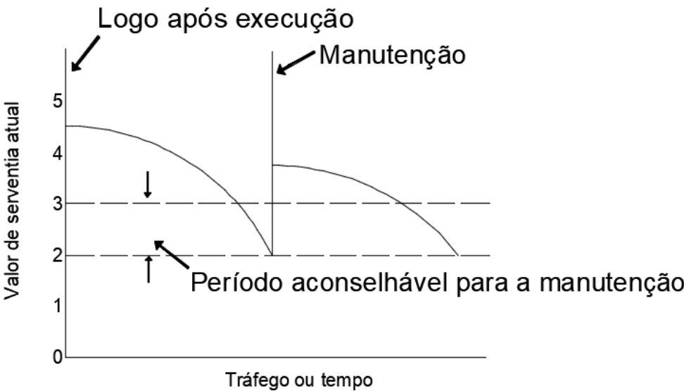
Figura 3: nível de serventia esperável Fonte: Os autores, adaptado de Bernucci et al. , (2008).
